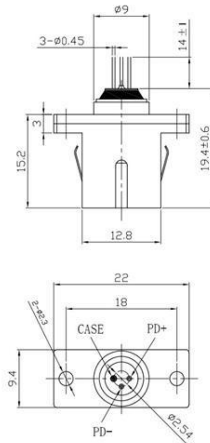
Fig1. SC Receptacle Module
